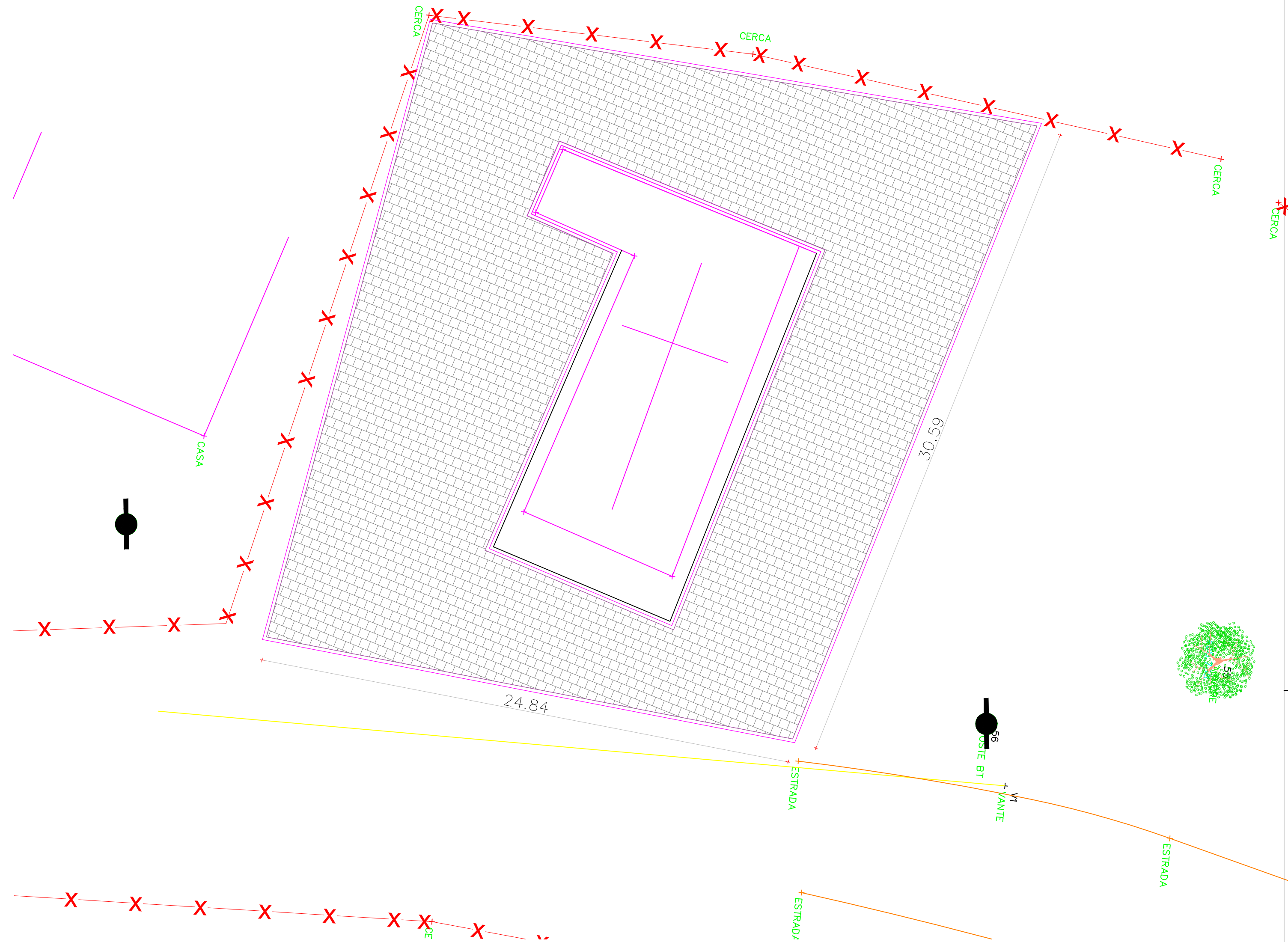
2 PAVIMENTAÇÃO ESCALA 1/150
