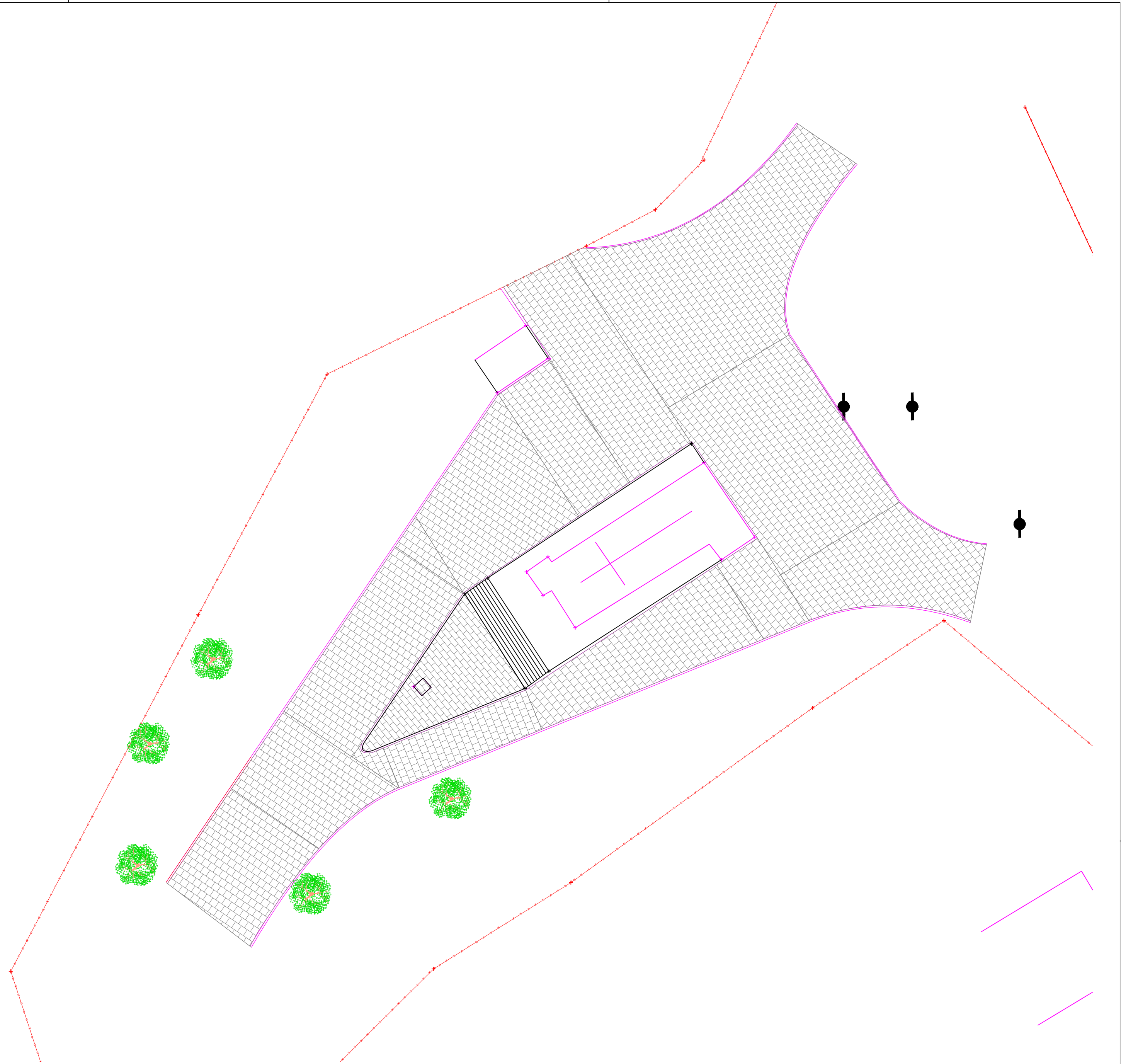
2 PAVIMENTAÇÃO ESCALA 1/150
